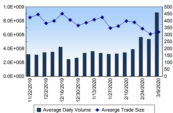
TSX Volume
